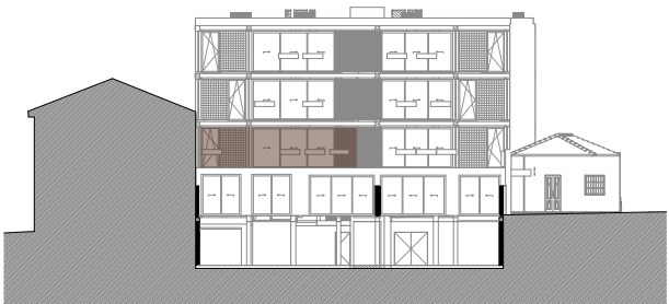
ALÇADO NASCENTE
