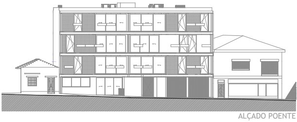
ALÇADO POENTE
