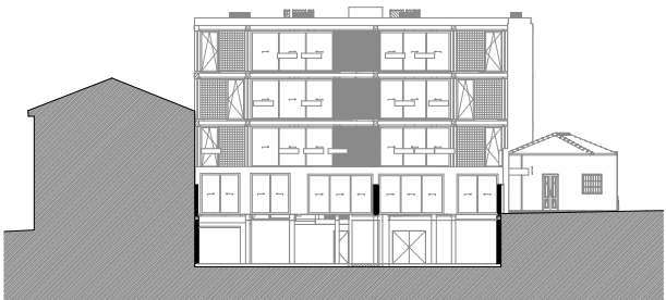
ALÇADO NASCENTE
